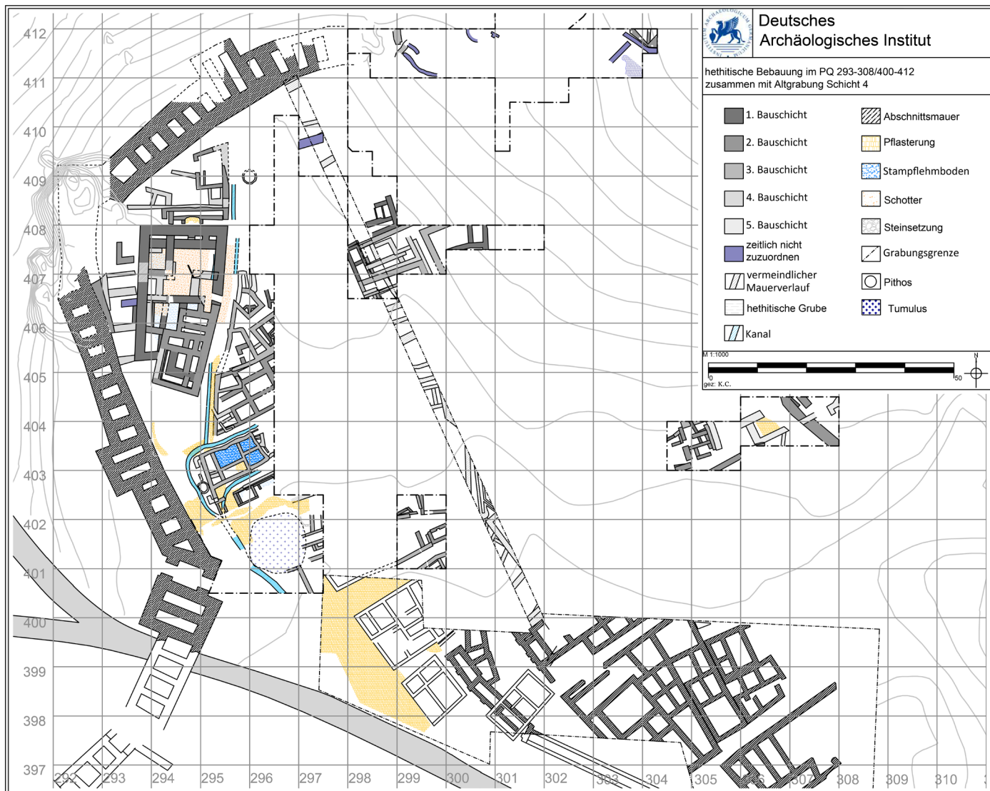
Boğazköy-Hattuša: Grabungen in der nördlichen Unterstadt, Stand 10/2020; erstellt von K. Czarnitzki auf Grundlage der Grabungsdokumentation (Boğazköy-Archiv des DAI, Istanbul)
